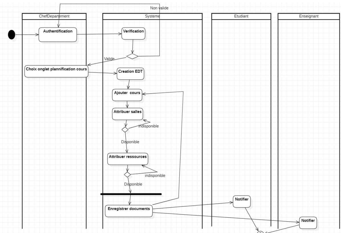
Figure 4: Diagramme d'activité
